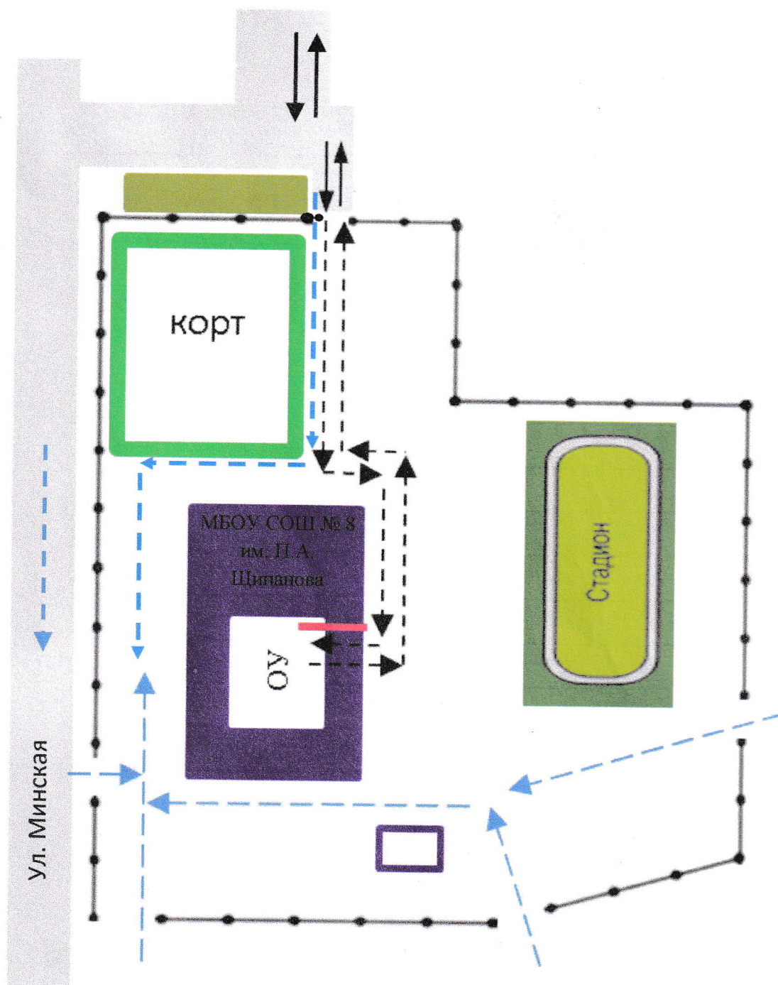
План-схема путей движения транспортных средств к местам разгрузки/погрузки и рекомендуемых путей передвижения детей по территории МБОУ СОШ № 8 им. П.А. Щипанова города Кузнецка
